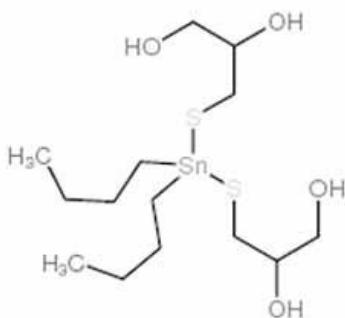
1- 硫代甘油 FASCAT 4224
